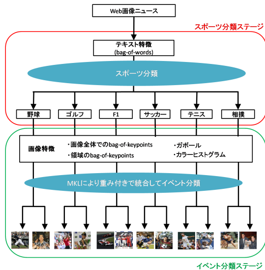
図 2 2段階手法の処理の流れ
