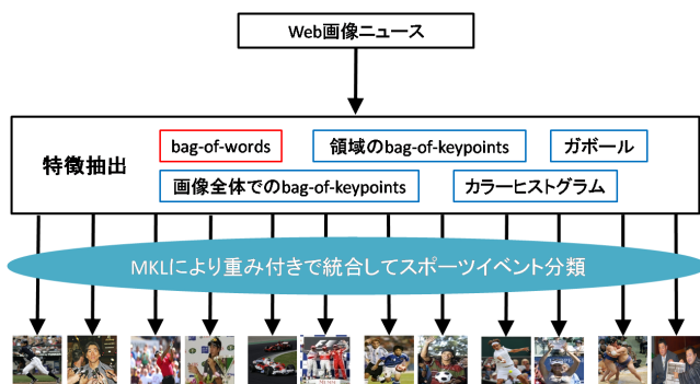
図 3 1段階手法の処理の流れ
